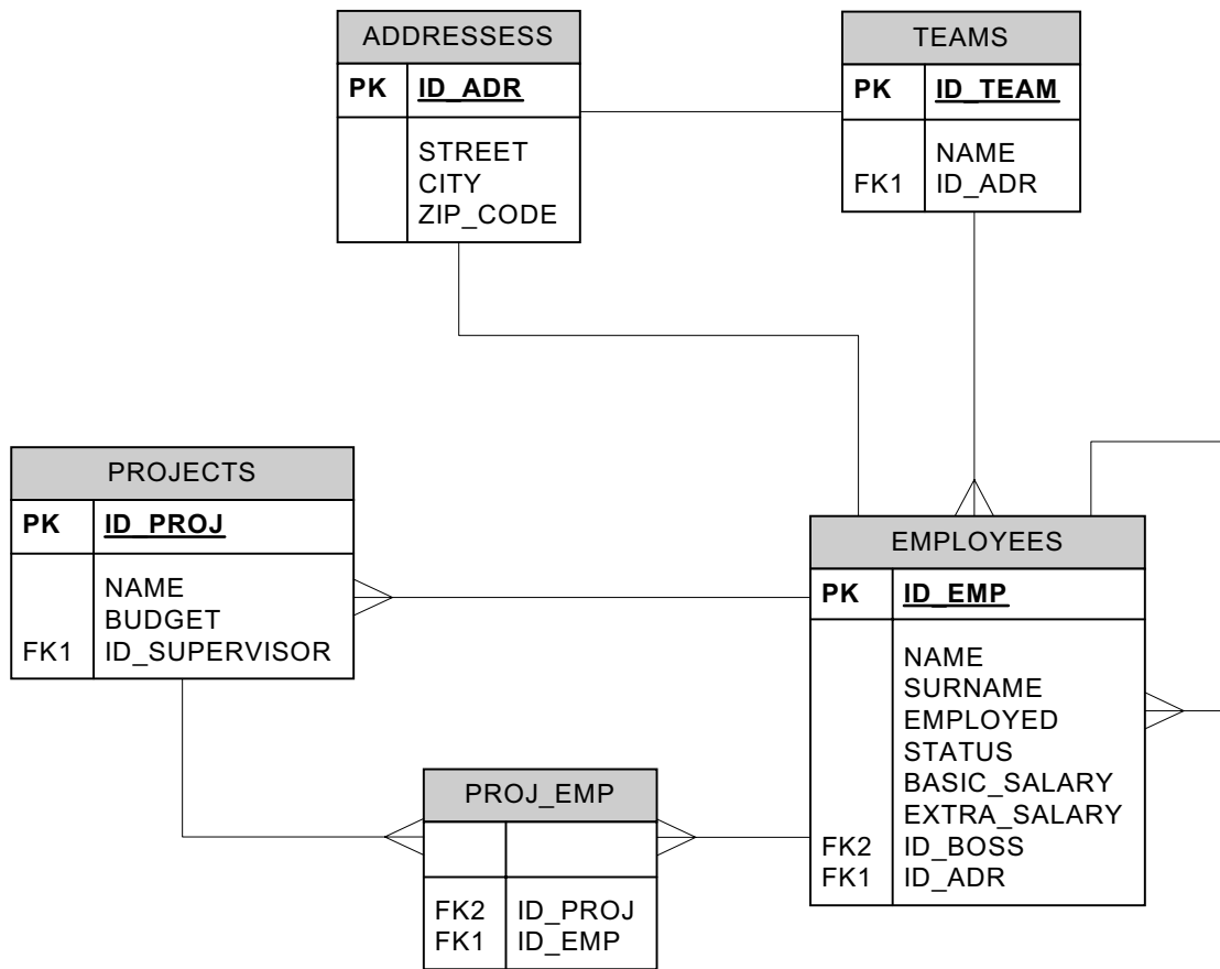
Rys. 1. Schemat relacyjnej bazy danych
