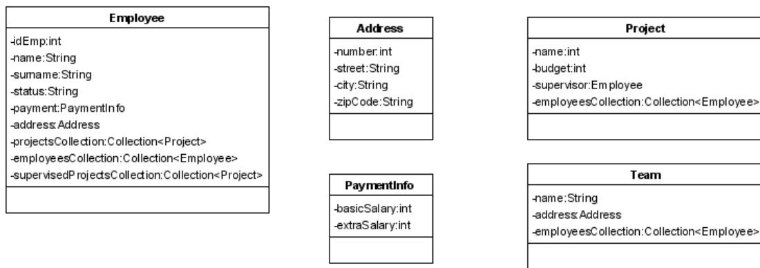
Rys. 2. Obiektowy model danych aplikacji
