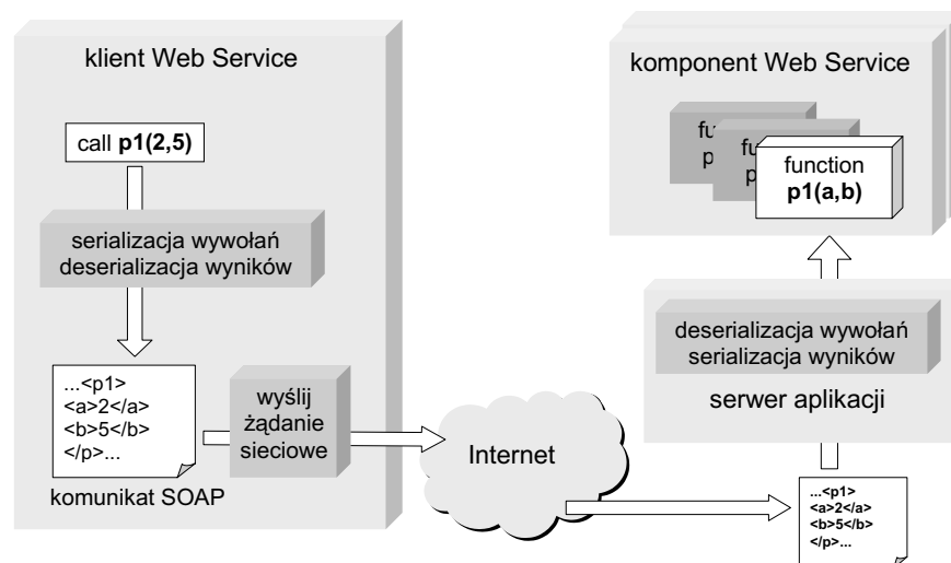
Rys. 2. Architektura wywołania komponentu Web Service
