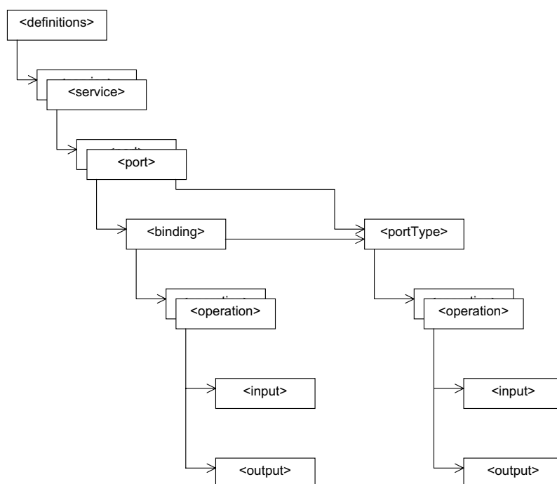
Rys. 6. Struktura znaczników dokumentu WSDL
