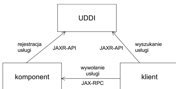
Rys. 10. Cykl życia usługi Web Service
